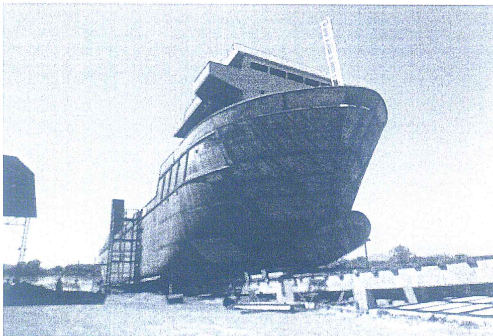
Status da construção - CASCO
